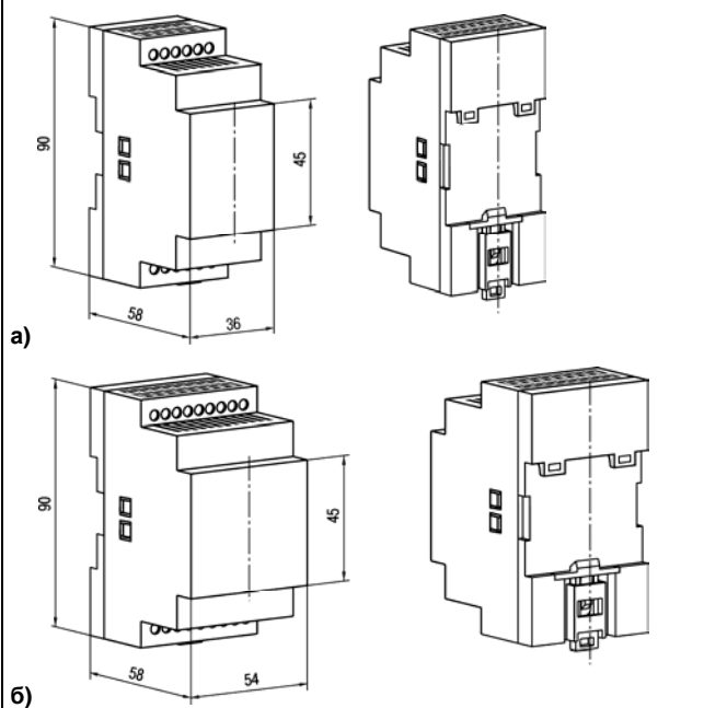
Рисунок 4.1 – Габаритные размеры блоков сетевого фильтра БСФ-Д2-0,6 (а) и БСФ-Д3-1,2 (б)
