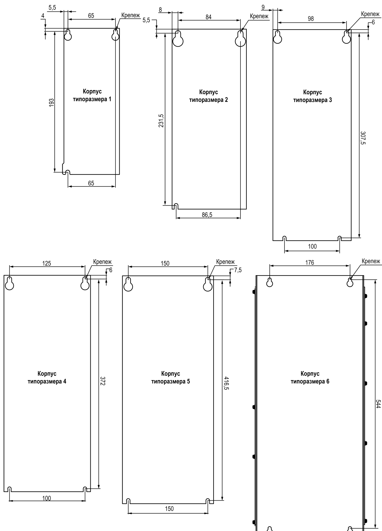
Рисунок 7.7 – Присоединительные размеры
