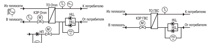
Рисунок 3 – Схема контура «ГВС»
