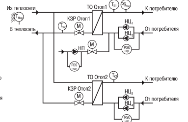
Рисунок 5 – Схема контура «Отопление + отопление»
