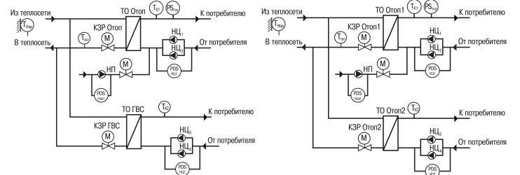
Рисунок 4 – Схема контура «Отопление + ГВС»
