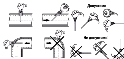
Рисунок 1 – Положения датчика при монтаже
