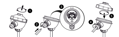
Рисунок 2 – Монтаж внешних электрических цепей
