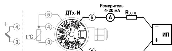
Рисунок 4 – Схема подключения
