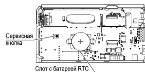
Рисунок 15 – Под лицевой панелью
